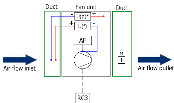
Fig. 5.4.2 VSVI EKO AL CPG fans
