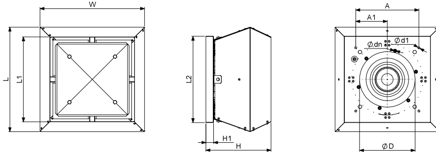
Fig. 4.2.9 VSV / VSV AL / VSV AL EKO
