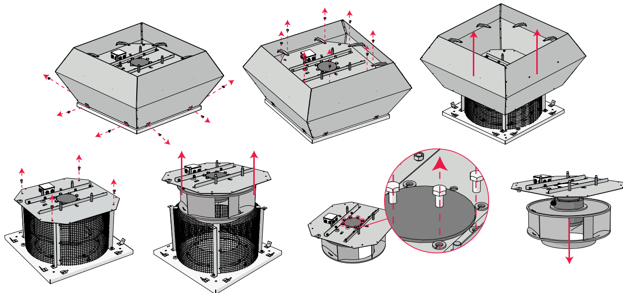
Fig. 6.4.6 VSV / VSV EKO / VSV EKO AL
