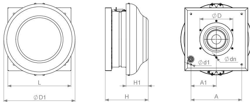
Fig. 4.2.8 VSA / VSA EKO
