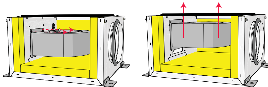
Fig. 6.4.1 AKU / AKU EKO
