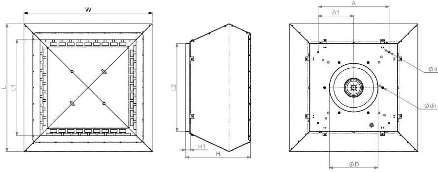
Fig. 4.2.10 VSVI / VSVI AL / VSVI AL EKO
