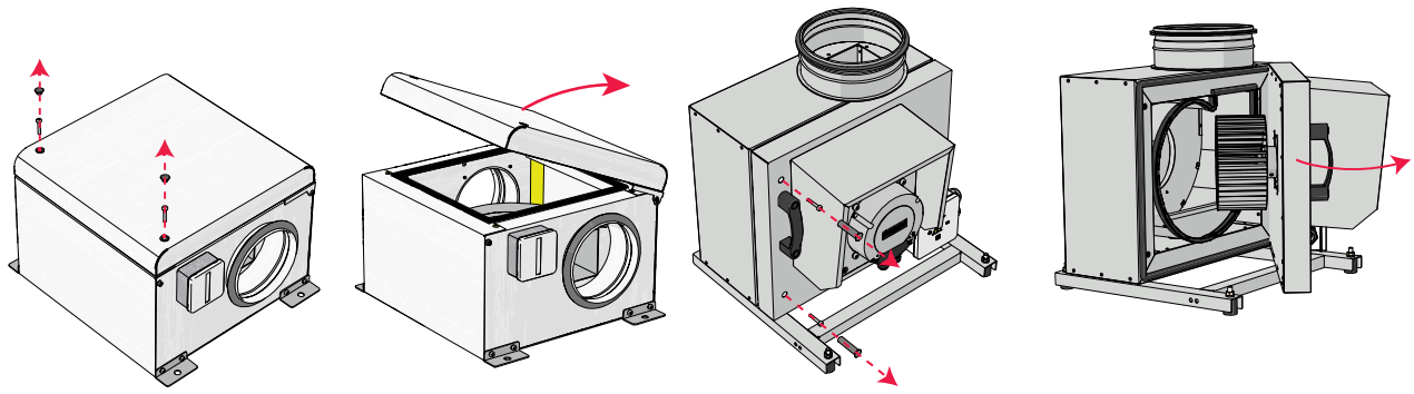
Fig. 6.3.1 AKU / AKU EKO
