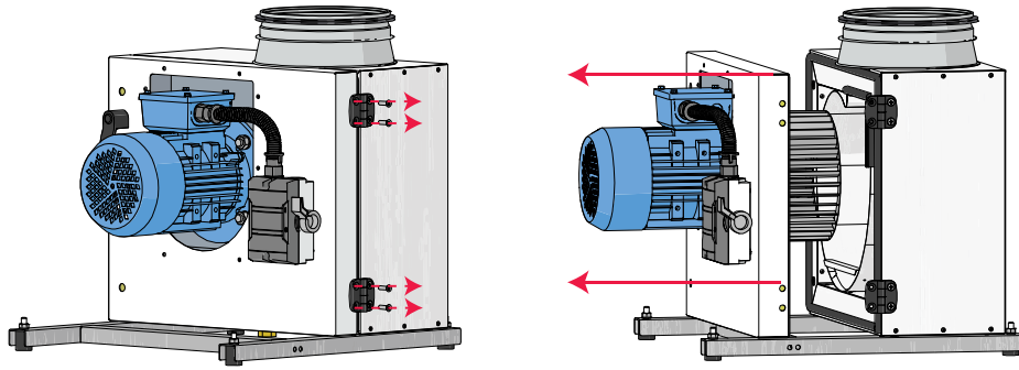
Fig. 6.4.2 KF T120 / KF T120 EC
