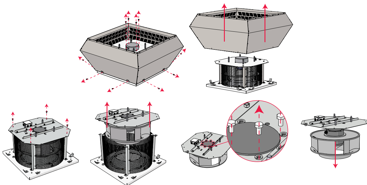
Fig. 6.4.7 VSVI / VSVI EKO / VSVI EKO AL
