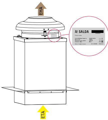
Fig. 2.10 VSA 3.0 / VSA EKO technical label place
